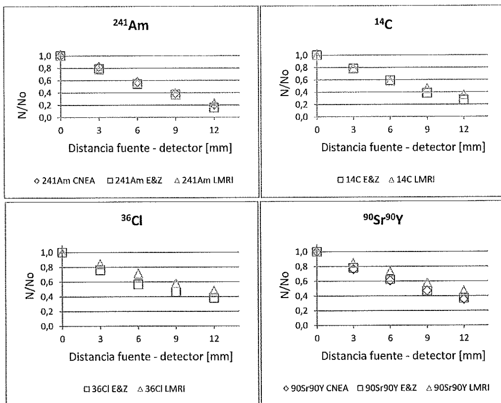
Figura 5. Flujo relativo de partículas (N/No) a 0 mm, 3 mm, 6 mm, 9 mm y 12 mm para las fuentes ^{241}\text{Am} , ^{14}\text{C} , ^{36}\text{Cl} y ^{90}\text{Sr}/^{90}\text{Y} .
