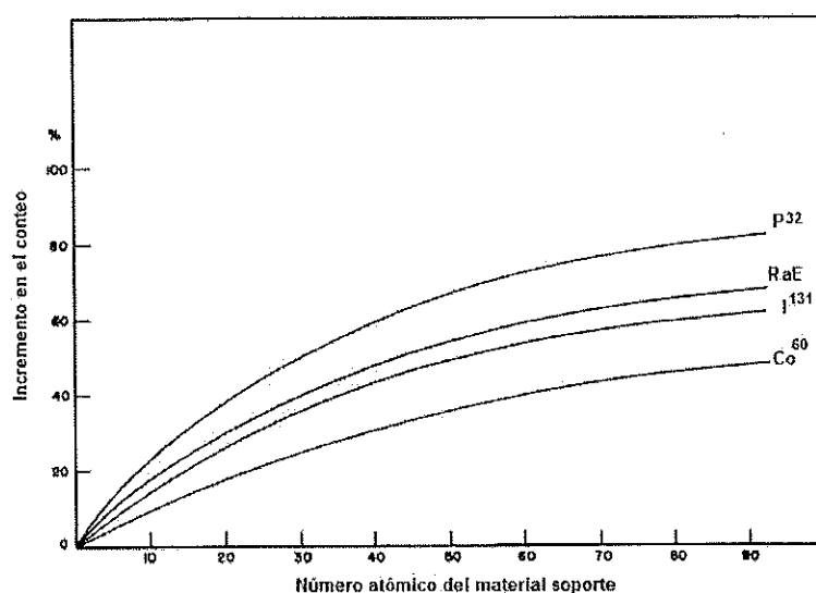
Figura 8. Incremento en el conteo de partículas por retrodispersión para varios radionucleidos en función del número atómico del soporte
